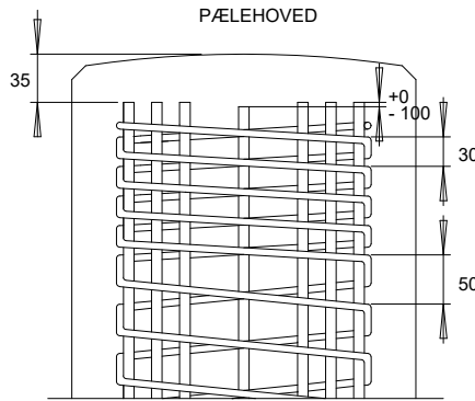
PÆLEHOVED
