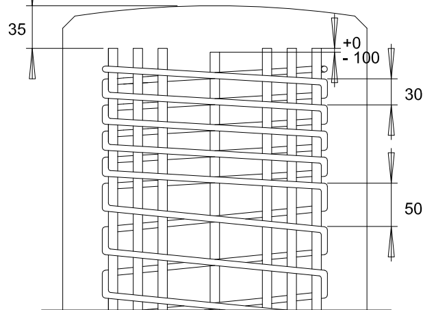
PÆLEHOVED
