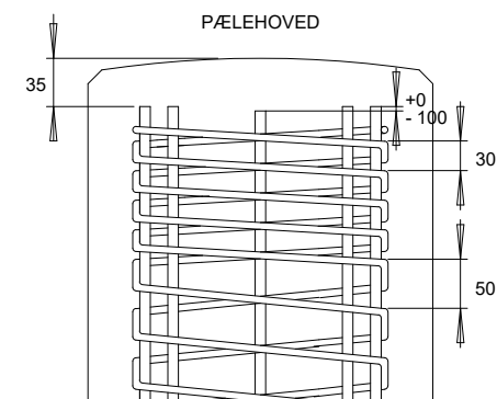
⑥ Forstærkningsbøjle ved pæleende
