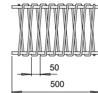
⑥ Forstærkningsbøjle ved pæleende
