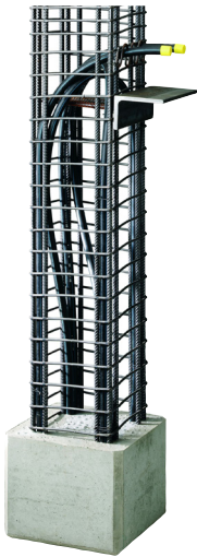
Energipælen er en traditionel funderingspæl opbygget i armeringsjern og beton, men med indstøbte jordvarmeslanger, hvori cirkulation af væske optager eller afgiver varme fra/til pælen og jorden.
